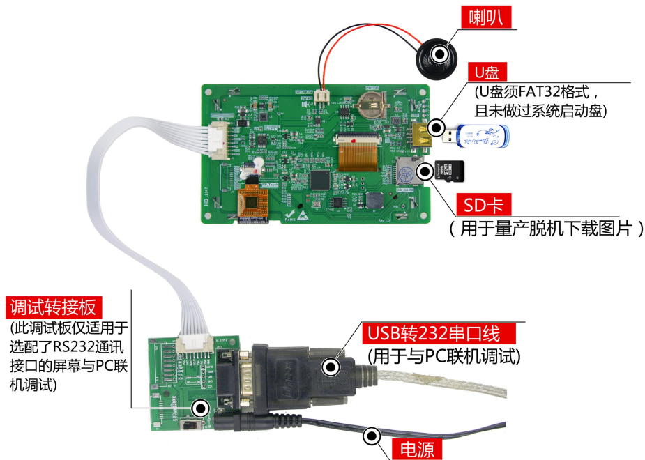
图 1-5 RS232 调试图
